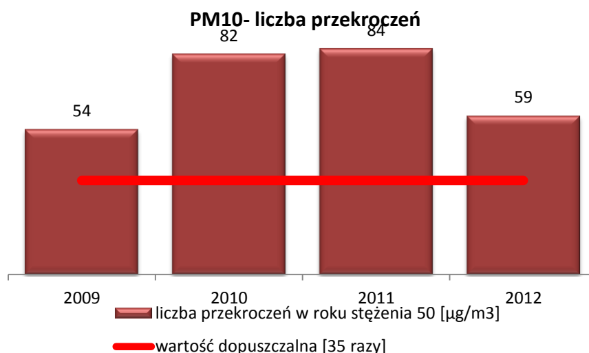
Rysunek 4. Liczba przekroczeń w roku dopuszczalnego stężenia dobowego na stacji pomiarowej w Mielcu w latach 2009-2012 20
