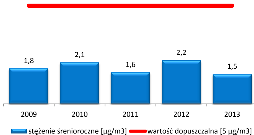
Rysunek 2. Stężenia średnioroczne benzenu na stacji pomiarowej w Mielcu w latach 2009-2013 18
