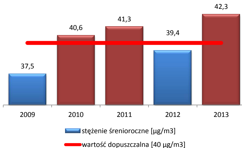
Rysunek 3. Stężenia średnioroczne pyłu zawieszonego PM10 na stacji pomiarowej w Mielcu w latach 2009-2013 19
